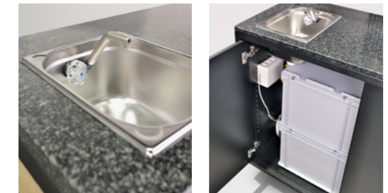
Integrierte Wasserversorgung Edelstahl-Waschbecken mit Wasserhahn für Bedientheke inkl. dezentraler Wasserversorgung mit Akkubetrieb 23 Liter Frischwassertank 23 Liter Abwassertank inkl. Türe mit Edelstahl-Beschlag Artikel-Nr.: 103562
